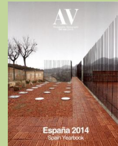
D(x) i
