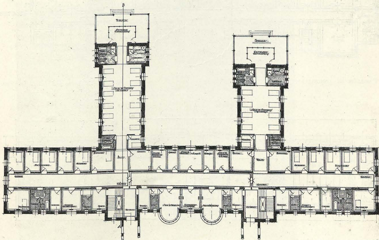
PLANO DE EMPLAZAMIENTO Y PLANTA BAJA DEL PABELLÓN DE CIRUGÍA.
