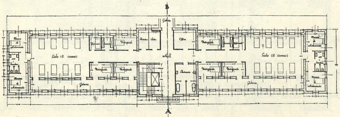
PLANTA DE UN PABELLÓN.
