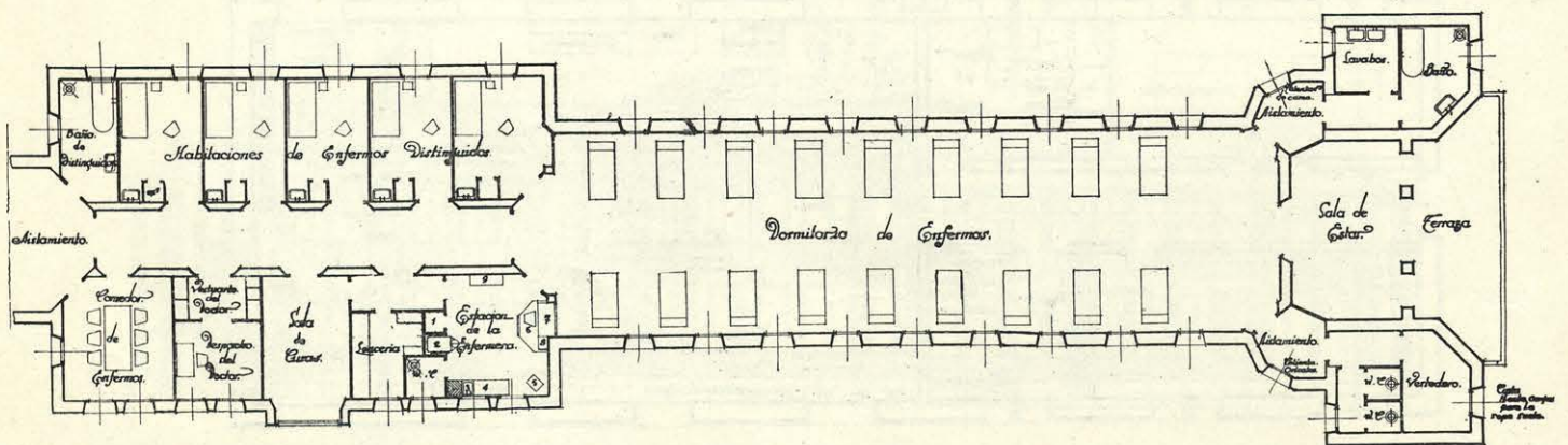
PABELLÓN DE CIRUGÍA.—PLANTA.
