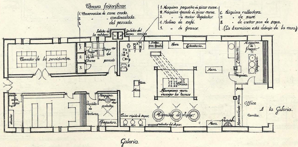
COCINAS: ALZADO Y PLANTA.
