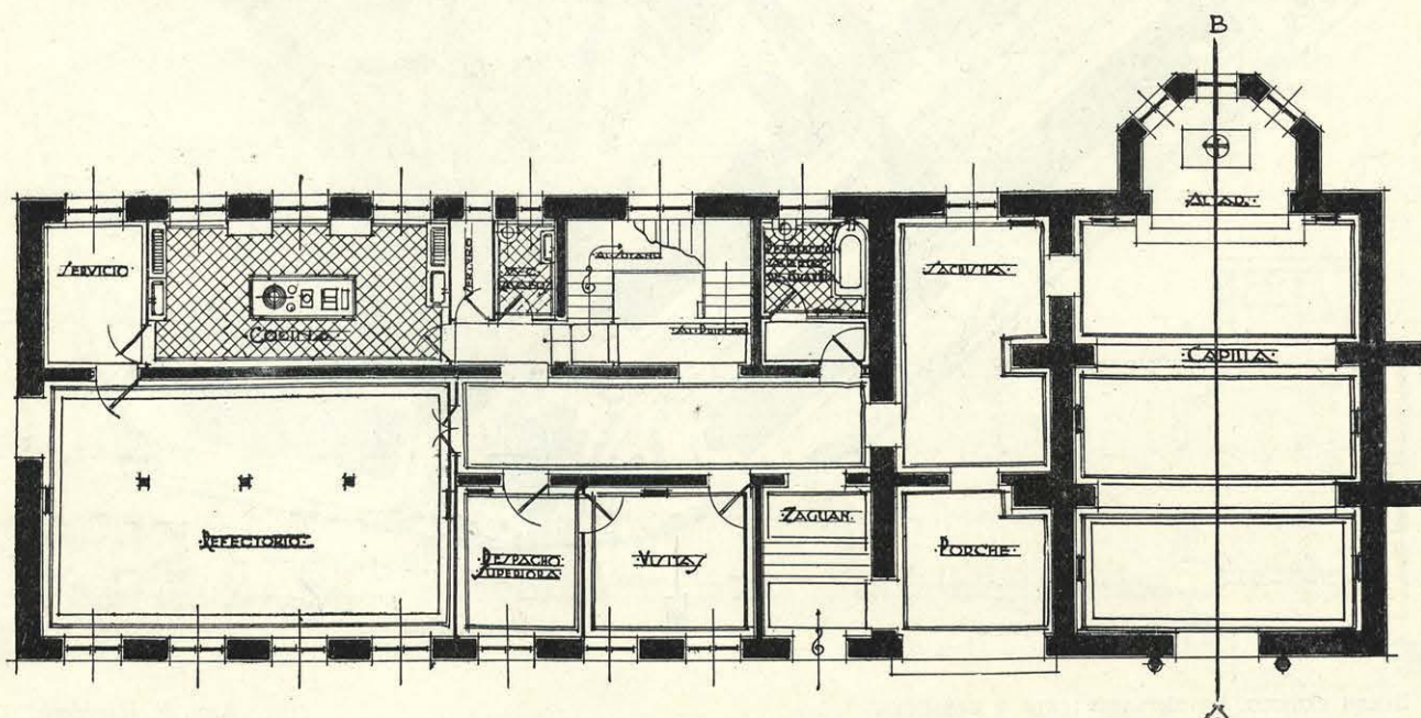
PABELLÓN DE HERMANAS.—PLANTA BAJA.
