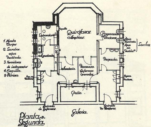
FACHADA LATERAL Y PLANTA DE QUIRÓFANOS.
