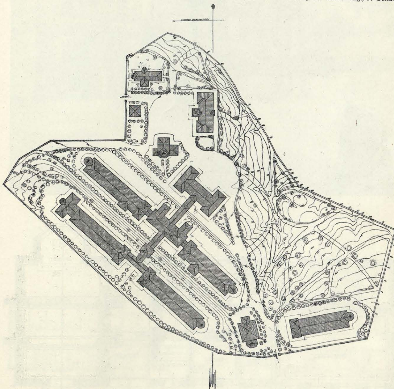
PLANO GENERAL DE EMPLAZAMIENTO Y DESAGÜES.
