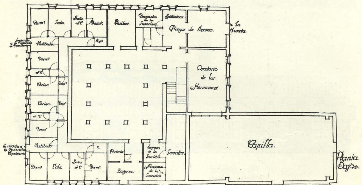
CONVENTO Y CAPILLA.—PLANTA BAJA
