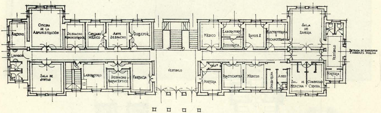
PABELLÓN DE ADMINISTRACIÓN.—PLANTA BAJA.
