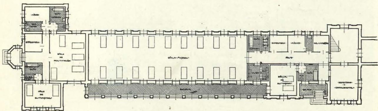
PLANTA DE UN PABELLÓN.
