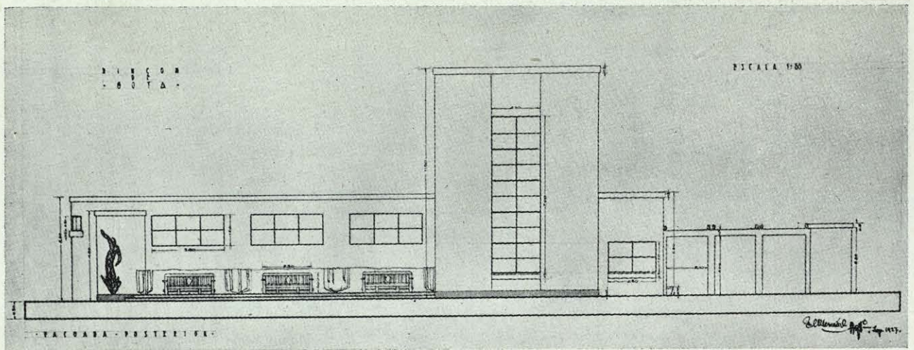
FACHADA POSTERIOR. (RINCÓN DE GOYA.)
