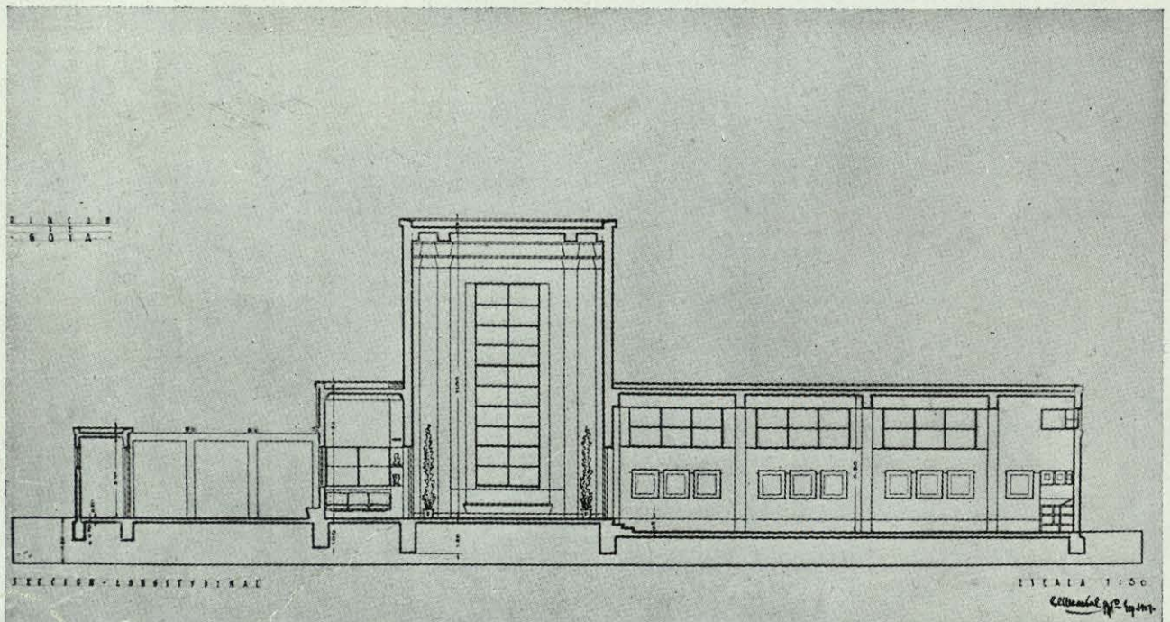
SECCIÓN LONGITUDINAL.
