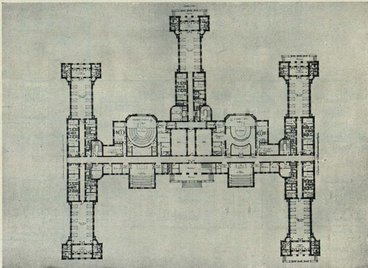
PLANTAS DE LOS PABELLONES MÉDICO (ARRIBA) Y QUIRÚRGICO (ABAJO).
