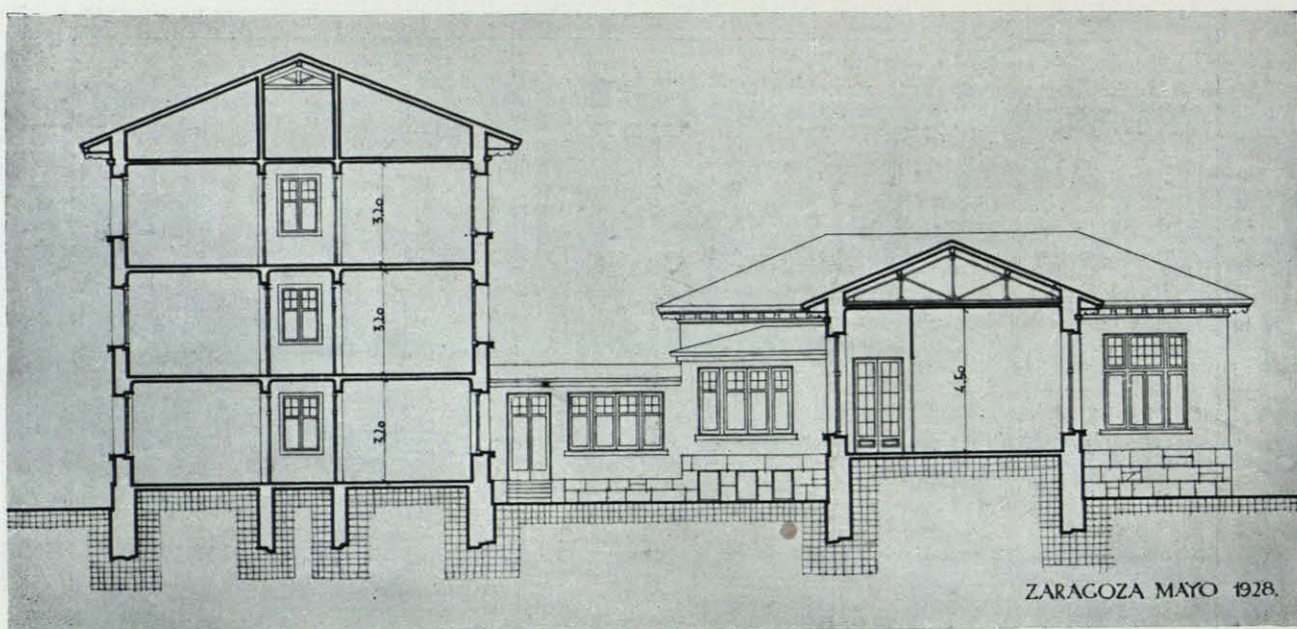
SECCIÓN DE LA RESIDENCIA DE ESTUDIANTES EN JACA.
