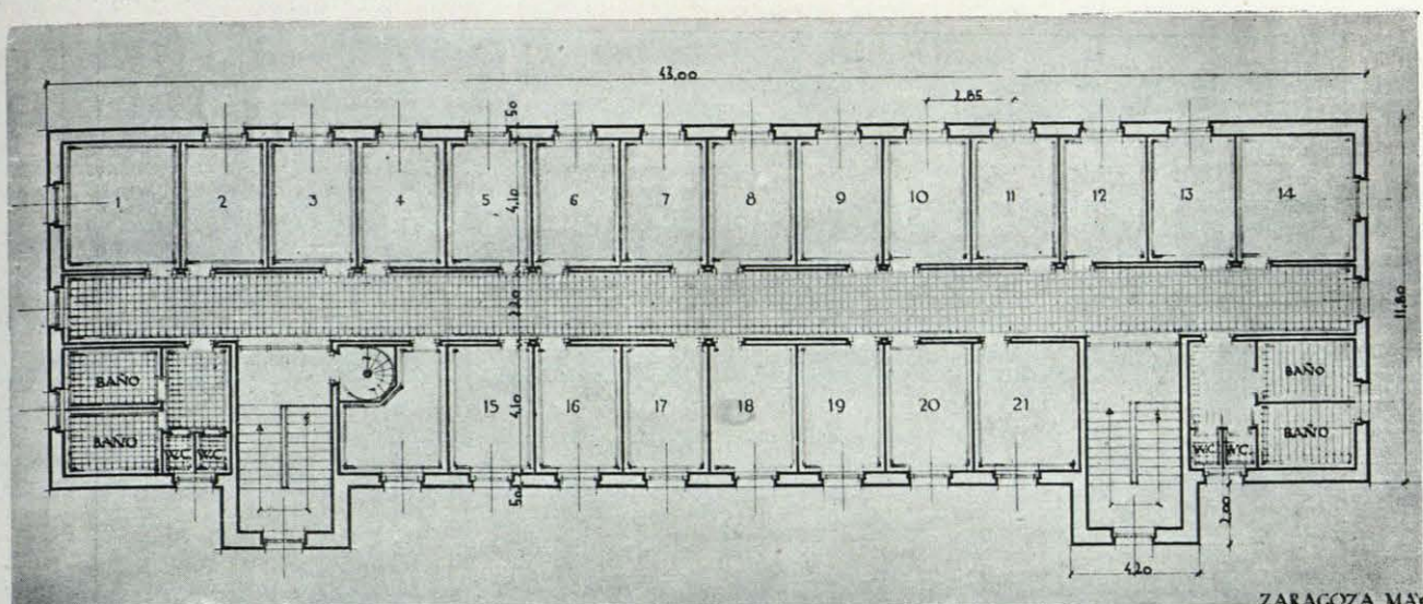
RESIDENCIA EN JACA. PLANTA DE DORMITORIOS.
