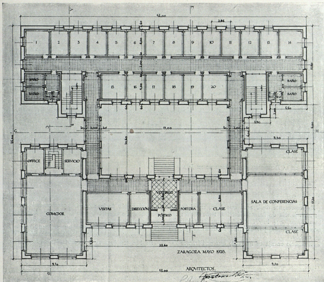
RESIDENCIA EN JACA. PLANTA.
