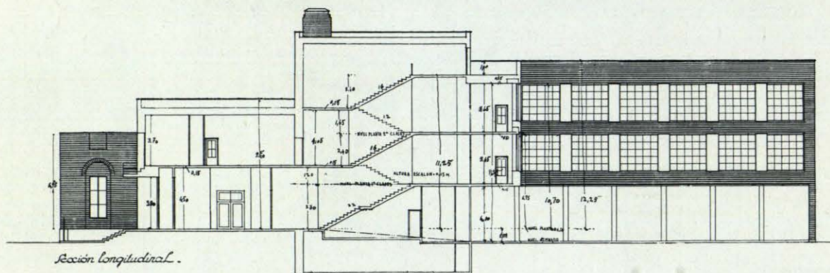
Secciones de la Sala de Conferencias.
