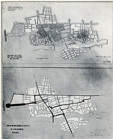
ELCHE. — PLANO ACTUAL DE LA CIUDAD Y PROYECTO DE REFORMA.
