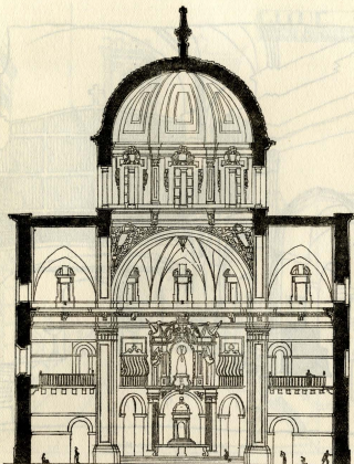
Elche. — Sección transversal de la iglesia de Santa María.
