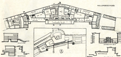
ARQUITECTO PROFESOR, OTTO BÜNZ.—PUERTO AÉREO EN BERLÍN.—PLANTA, SECCIONES Y PERSPECTIVA GENERAL.
