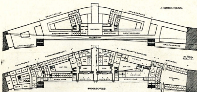
ARQUITECTO PROFESOR, OTTO BÜNZ.—PUERTO AÉREO EN BERLÍN.—PLANTAS DE LOS EDIFICIOS.
