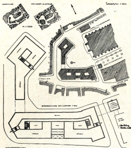
PROYECTO PARA LA MÜNSTERPLATZ DE ULM.—PLANTAS DE EMPLAZAMIENTO Y DE DETALLE.
