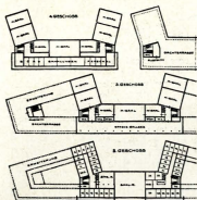
ARQUITECTO PROFESOR, OTTO BÜNZ.—PUERTO AÉREO EN BERLÍN.—PLANTAS Y DETALLES.
