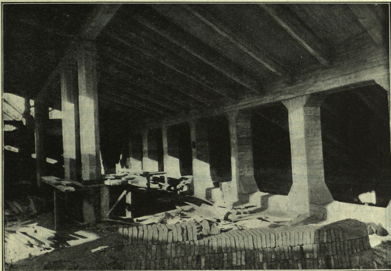
Piso del «foyer» y anfiteatro de hormigón armado con viga «Vierendeel» de 22 metros de luz.
