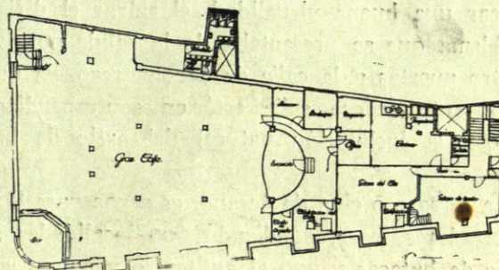
PLANTA DE SÓTANOS
