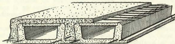
FIG. 1.ª—SECCIÓN DE UN SUELO GEF.
