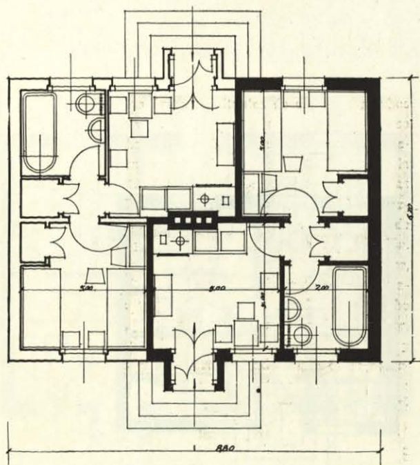
BLOQUE DE DOS VIVIENDAS CONSTITUIDAS POR UNA COCINA-COMEDOR, UN DORMITORIO, CUARTO DE BAÑO Y ROPEO.
