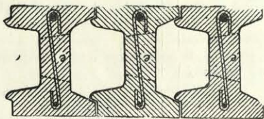
FIG. 3. a —SECCIÓN DE UN SUELO HALLER.
