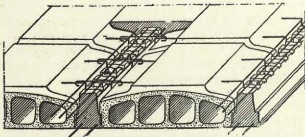
FIG. 5. a —SECCIÓN DE UN SUELO SISTEMA PLANCHE.
