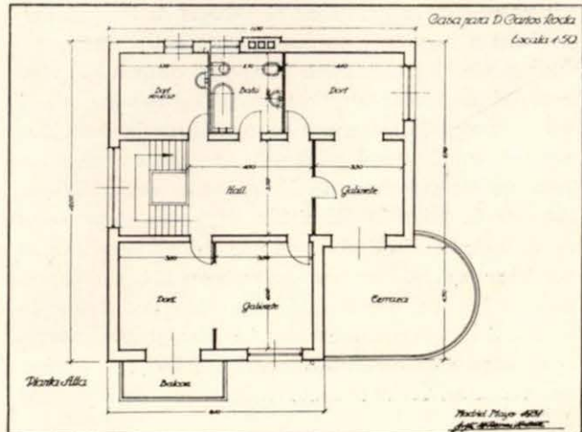
CASA PARTICULAR (MADRID) ARQ., J. M. RIVAS EULATE
