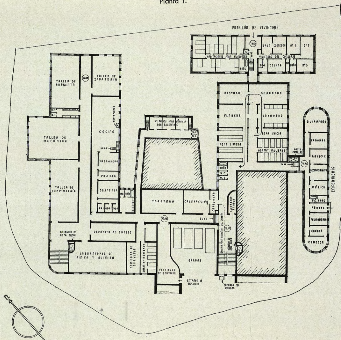
Planta 1.
