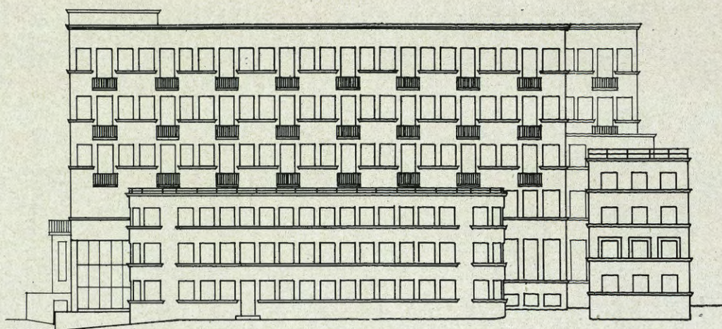
FACHADA S-E
