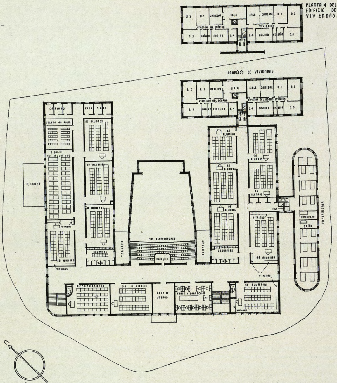
Planta 3.
