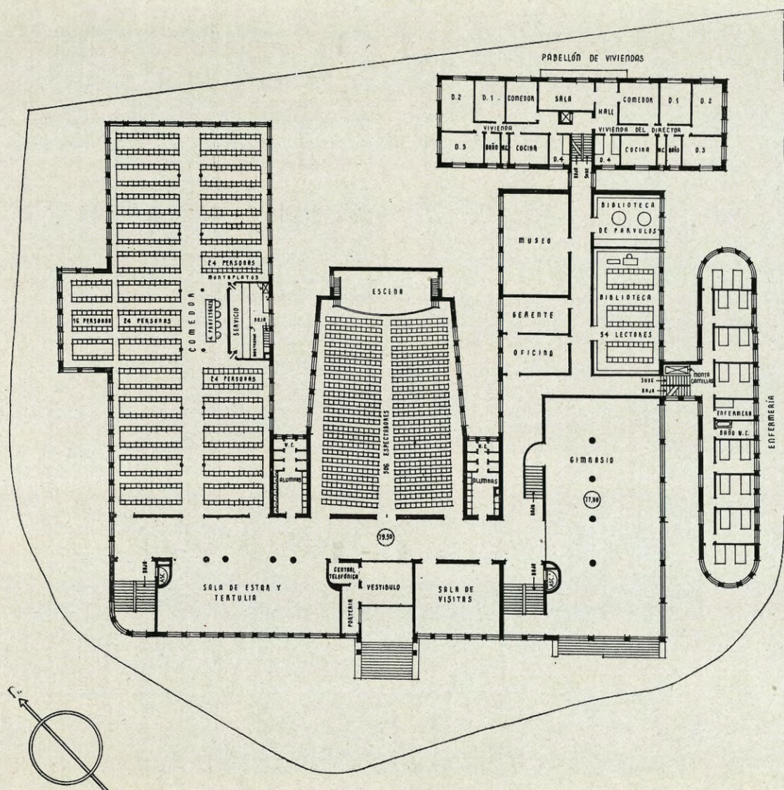
Planta 2.
