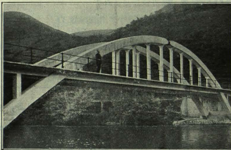
Puente del Dáneo (Asturias), en hormigón armado, de 42 metros de luz. - Articulación única en la clave. - Arcos sin ningún arriostramiento superior. - Ejecutado exclusivamente con CEMENTO TUDELA-VEGUIN
