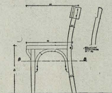
COSTADO
