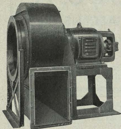
Ventilador centrifugo para grandes caudales.
