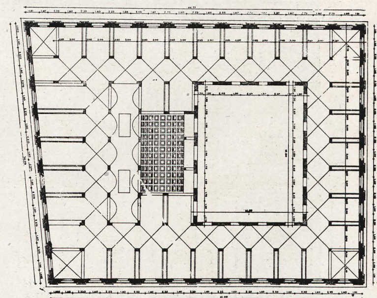
Plantas de la Delegación de Hacienda de Alicante (Primer premio).
