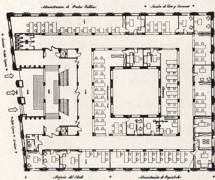
Plantas de la Delegación de Hacienda de Alicante (Primer premio).
