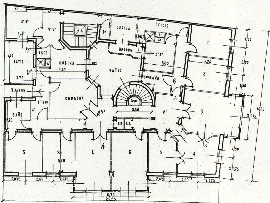
Planta general de pisos.
