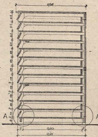
SECCION
