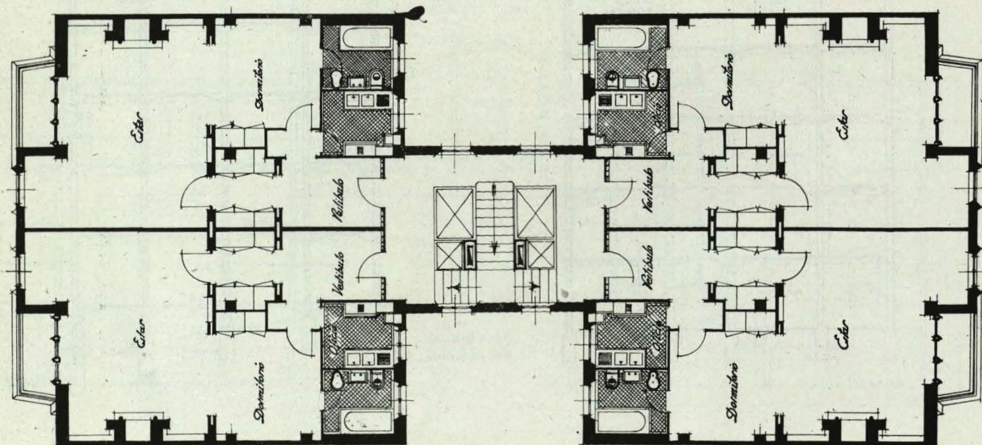
Pormenor de la fachada y del interior y planta normal de pisos.
