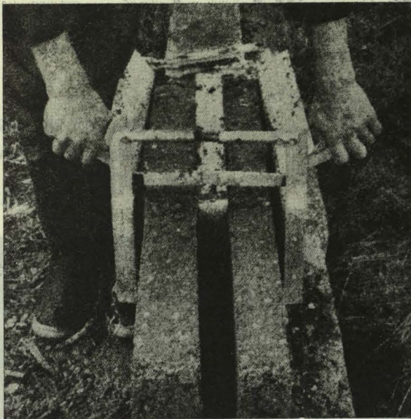
El fraguado casi inmediato del hormigón empleado permite soltar la gabera y deslizarla horizontalmente.
