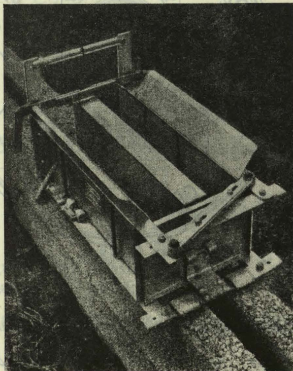
La gabera metálica corrediza para muros de hormigón.
