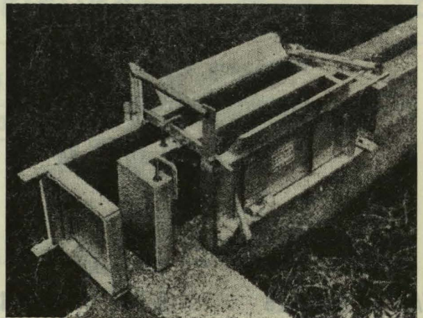
Pieza especial de esquina que se acopla al elemento normal.
