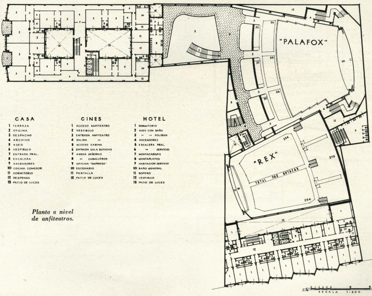
Planta a nivel del patio de butacas.
