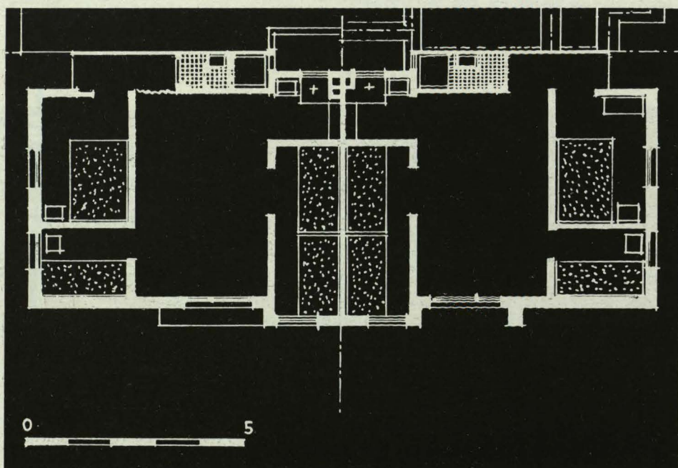
Planta de viviendas en galería.
