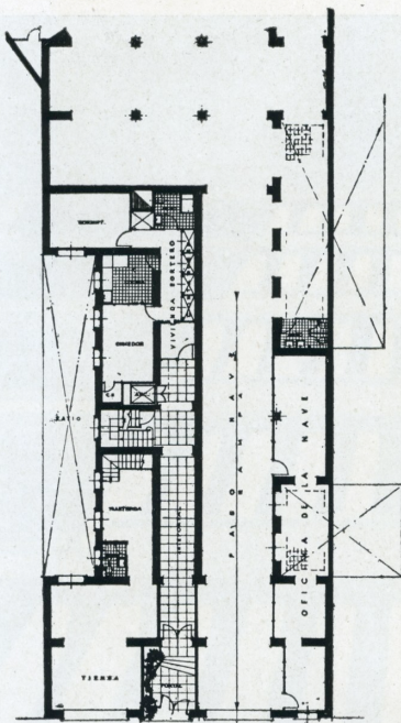
Planta baja.
