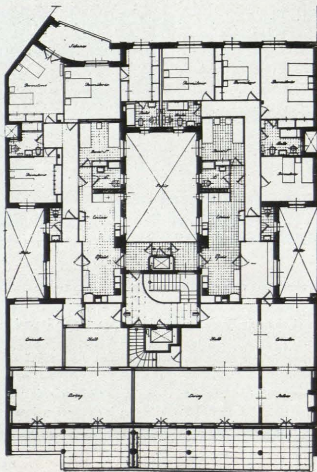
Planta de pisos.
