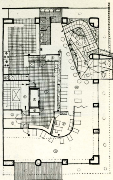
Plantas baja y alta y detalles de la instalación.
