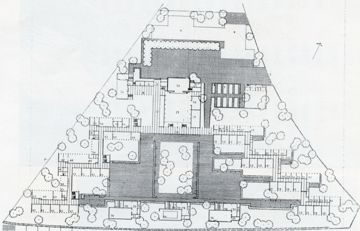
PLANTA DE CONJUNTO: 1. Entrada al centro cívico y a las escuelas; 2. Administración; 3. Aparcamiento de bicicletas; 4. Aparcamiento de coches; 5. Cine; 6. Biblioteca.—CENTRO CIVICO: 7. Entrada; 8. Club y salón de exposiciones; 9. Sala de lectura; 10. Cocina; 11. Salón de reuniones; 12. Guardarropas; 13. Teatro; 14. Escenario; 15, 16, 17 y 18. Anejos del teatro.—ESCUELA PRIMARIA: 19. Clases; 20. Comedores; 21 a 34. Servicios generales de la escuela.—GIMNASIO: 35. Vestuario; 36. Gimnasio; 38. Duchas; 39. Sauna; 40. Piscina.—ESCUELA SECUNDARIA: 41. Clases; 42. Auditorio; 43 a 53. Servicios anejos a la escuela; 54. Campos de juego.
