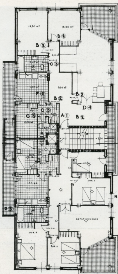
Planta tipo.
