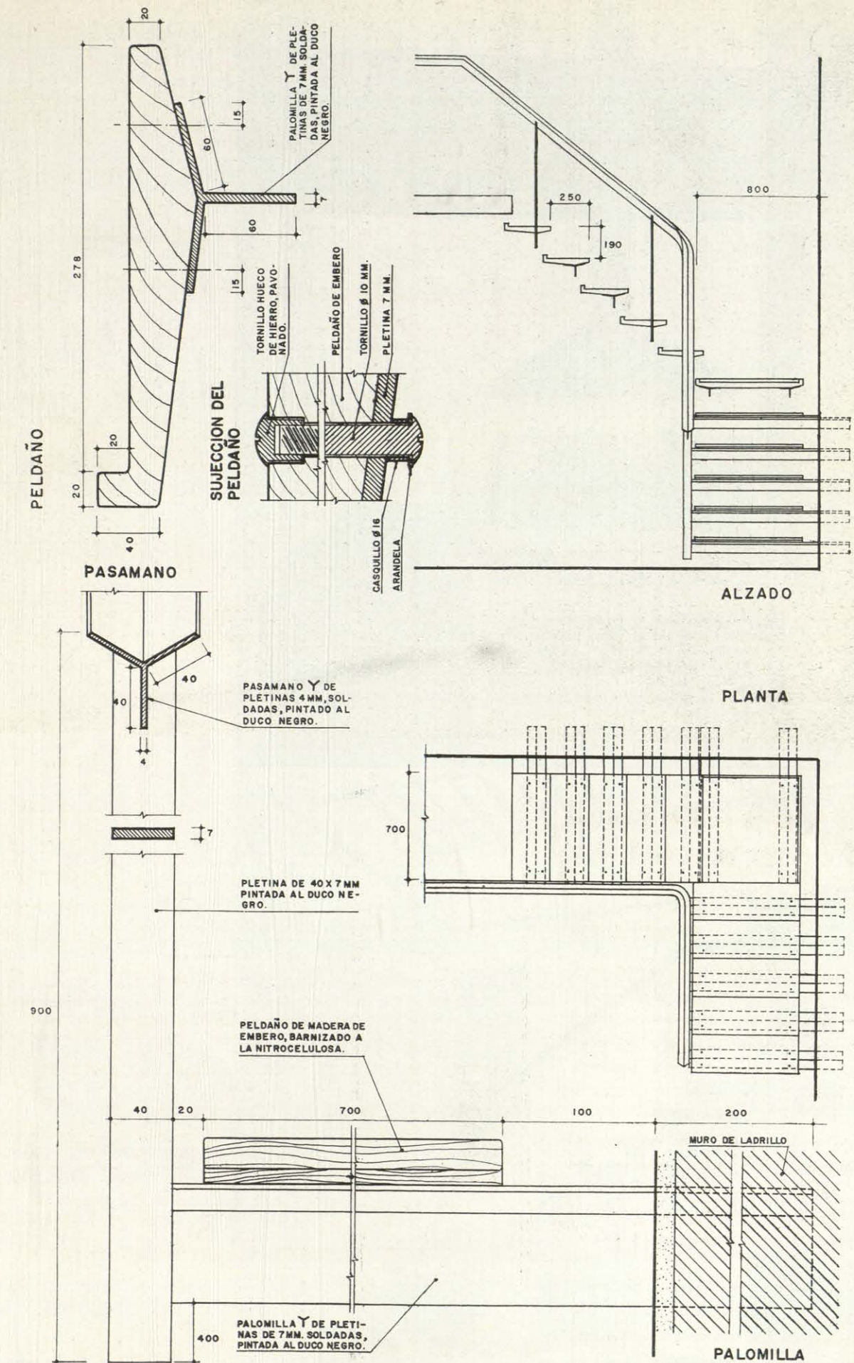
Detalle de la escalera.
