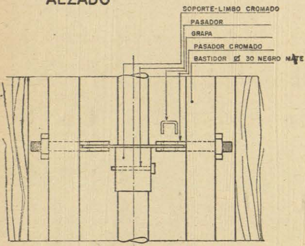
DETALLE 5
