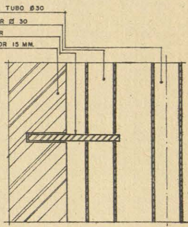
SECCION DEL DETALLE 6
