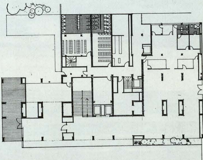
Planta baja.
