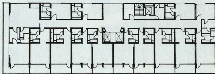
Planta tipo.
