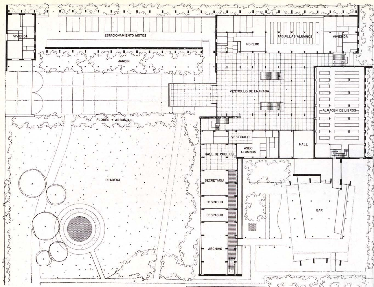
Planta baja.
