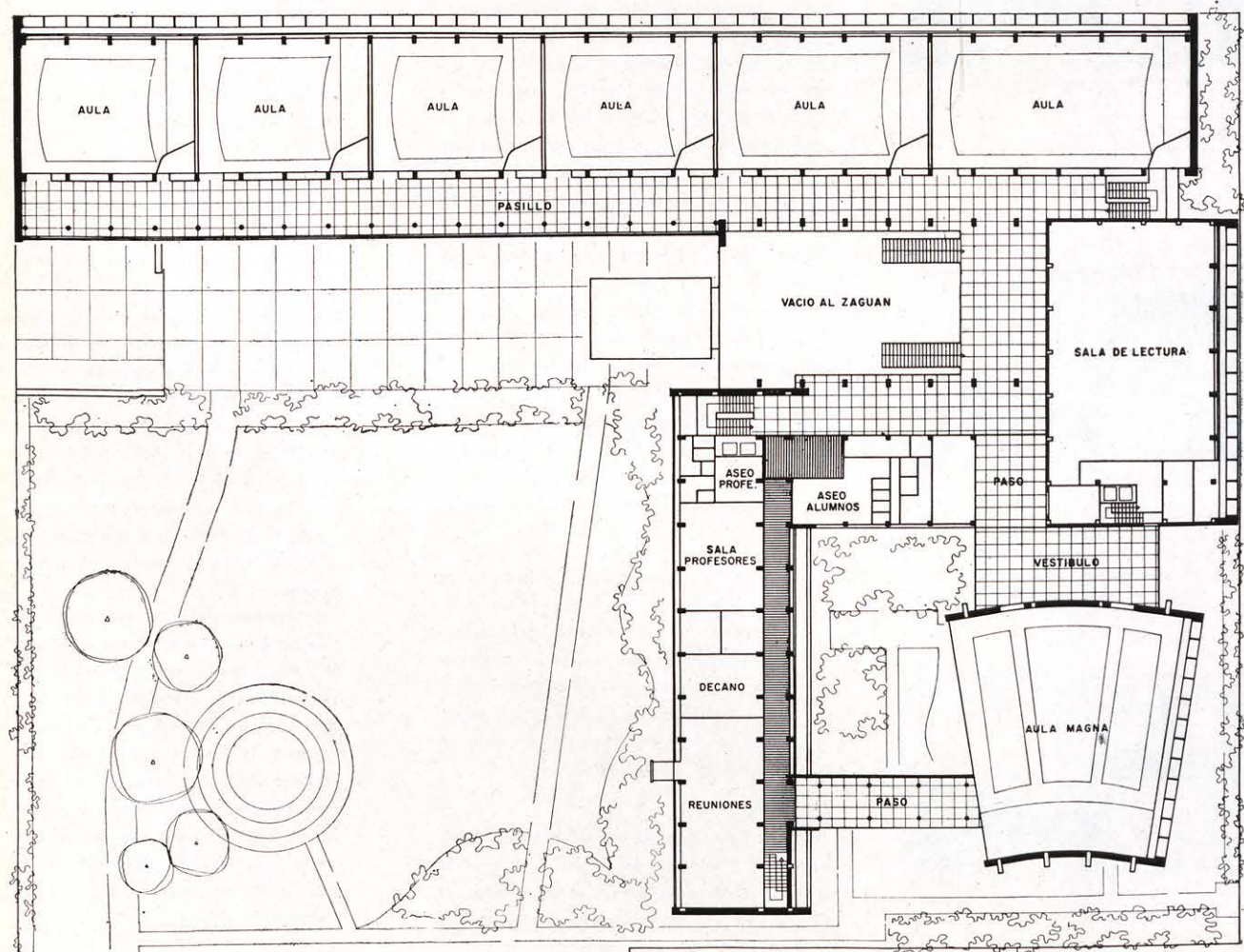
Planta primera.
