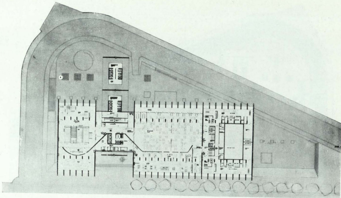
Planta semisótano ( — 1,70 — 2,30 )
