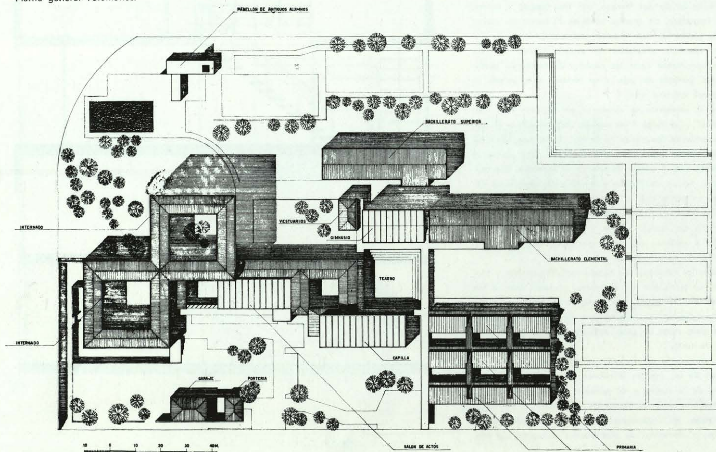
Planta general volúmenes.
