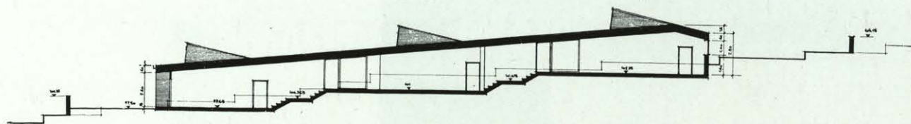
Alzado Sección.
