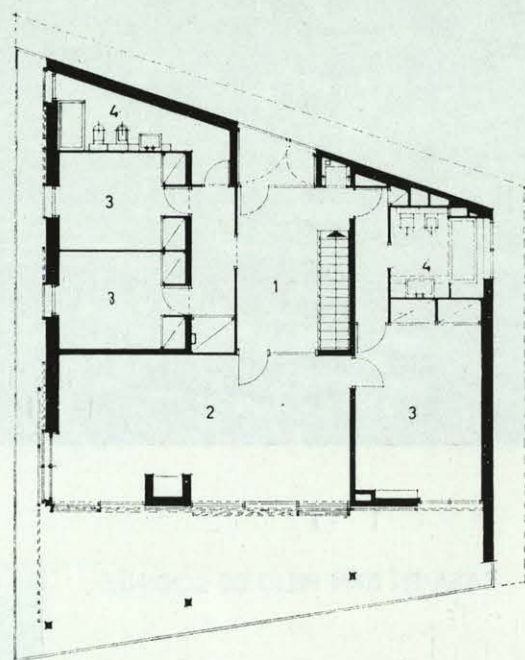
planta piso
