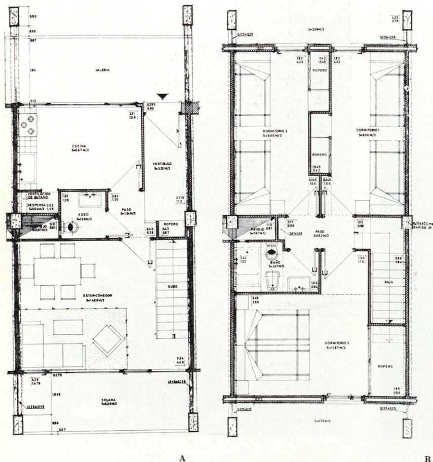
Planta tipo de pisos.
