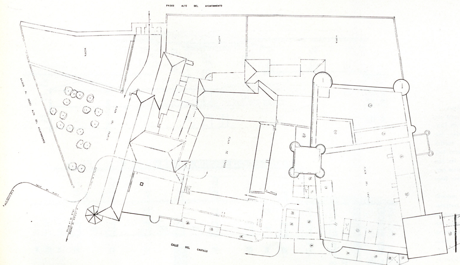
Planta de conjunto del Parador de Oropesa.
