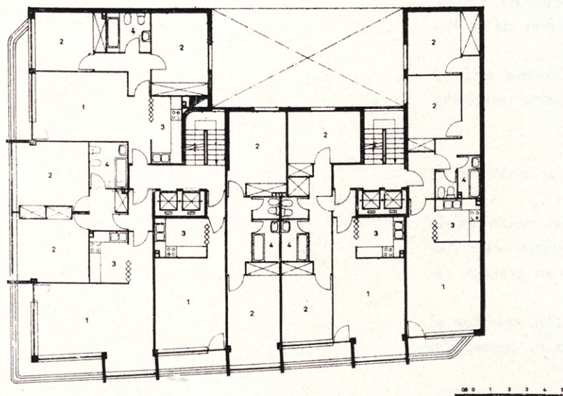
1. Cuarto de estar-comedor.—2. Dormitorio.— 3. Cocina.—4. Baño.
