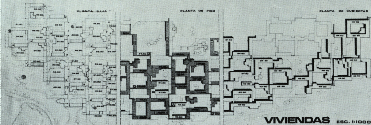
PLANTA BAJA
