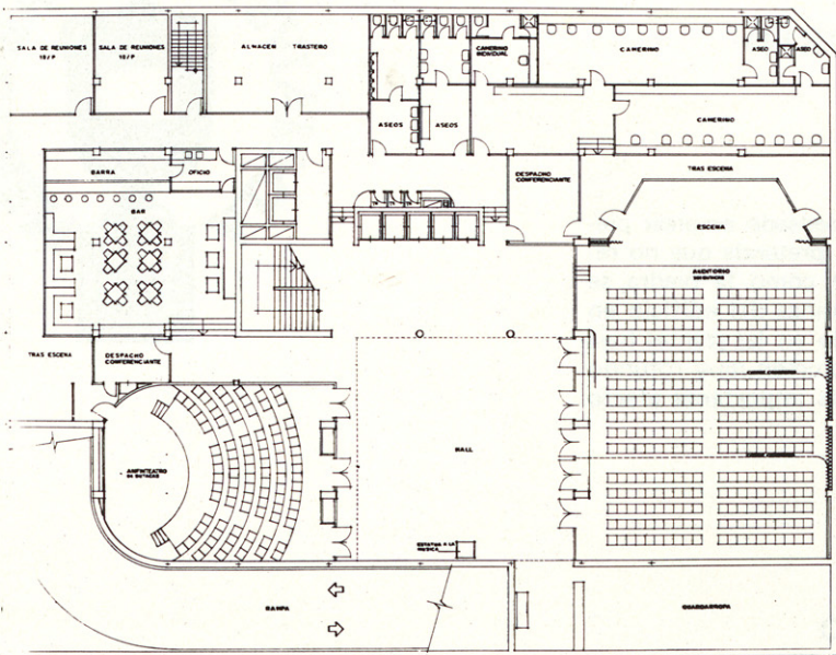
Planta 1er sótano
