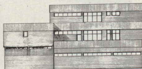
ALZADO OESTE
