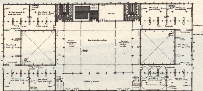
Planta Baja
