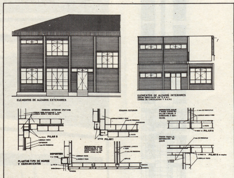
Detalles de fachada
