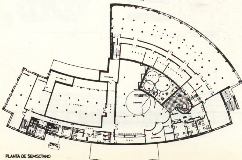
PLANTA DE SEMISOTANO
