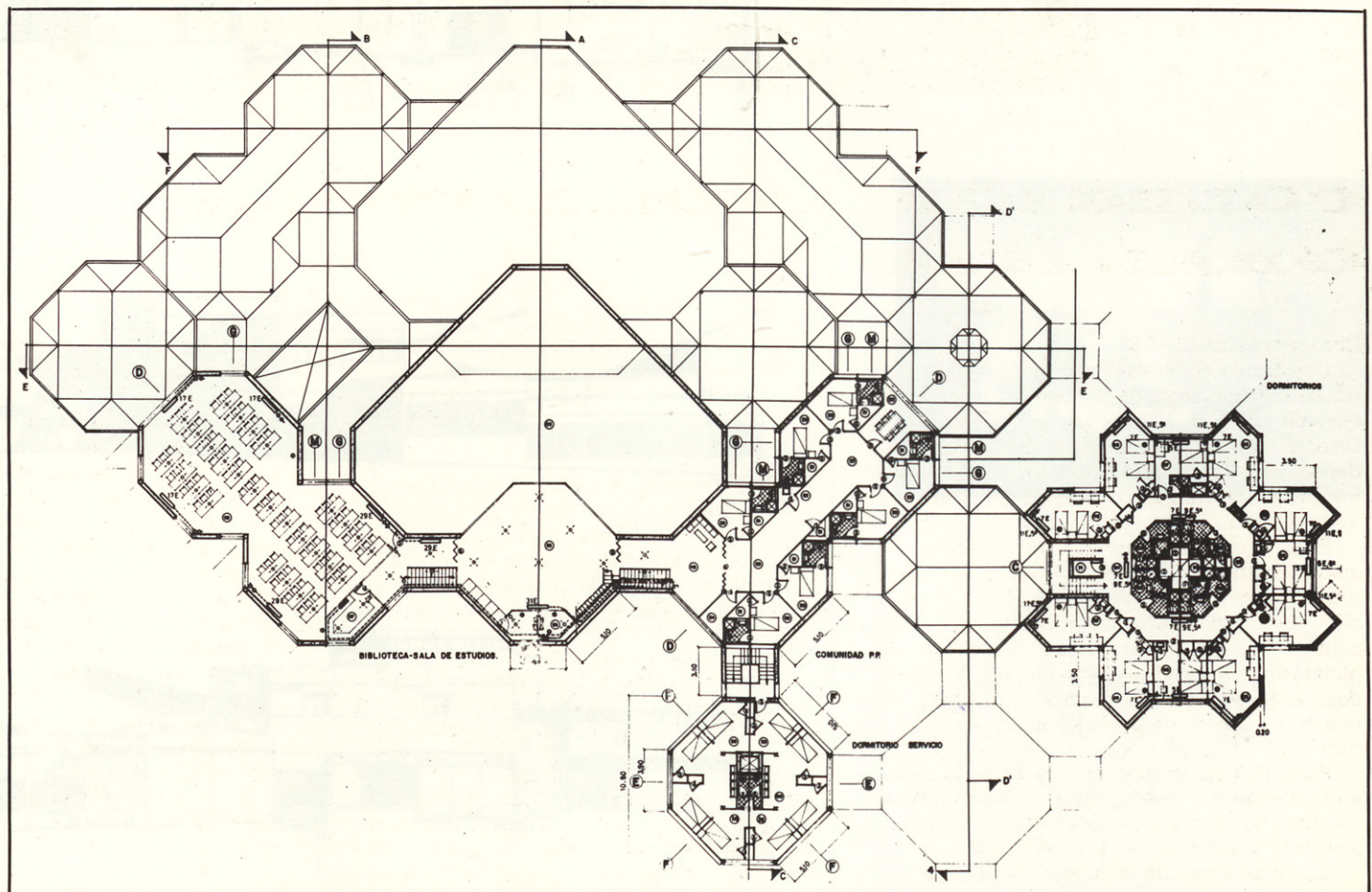
PLANTA PRIMERA
