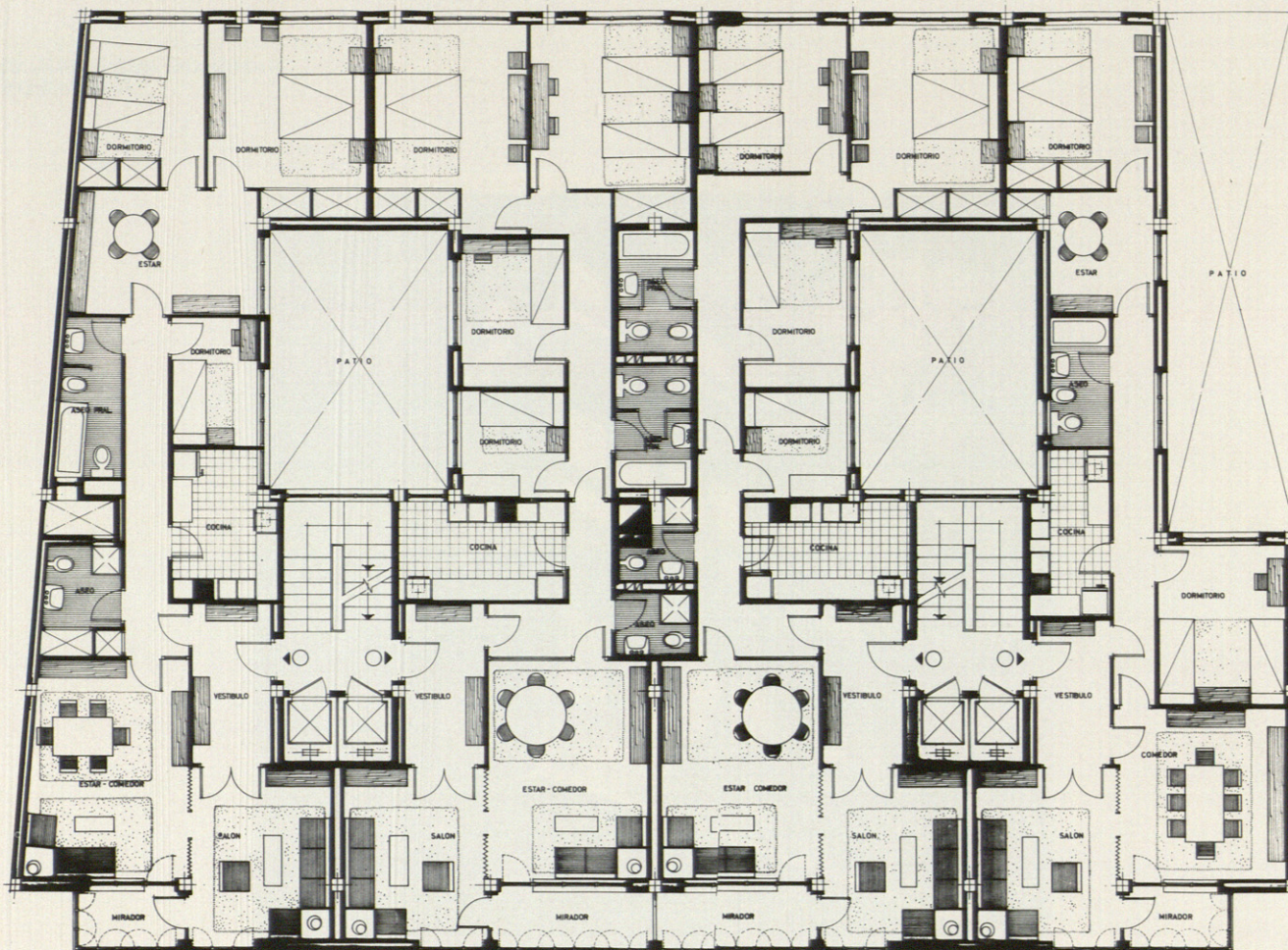
PLANTA TIPO
