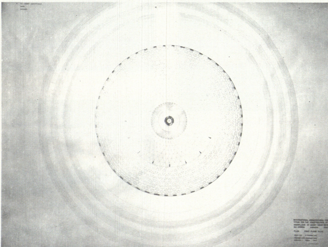
Monumento a Alí Jinnah, Pakistán. Planta.
