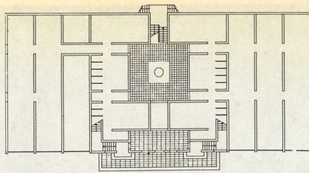
PLANTA BAJA
