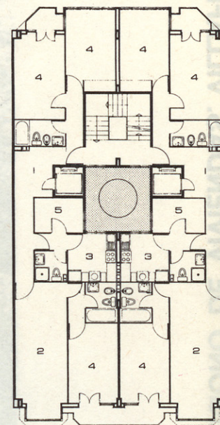
Planta 6.ª
