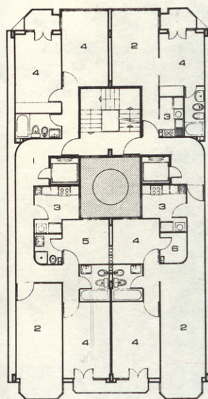
Planta tipo.
