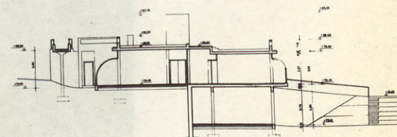
SECTION D-D
