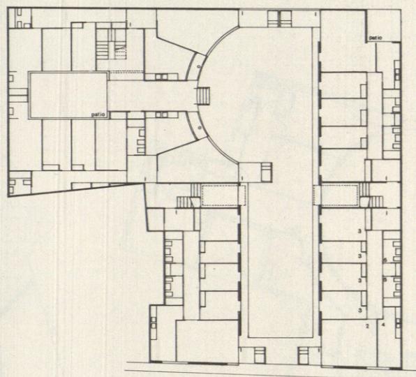
Planta baja.
