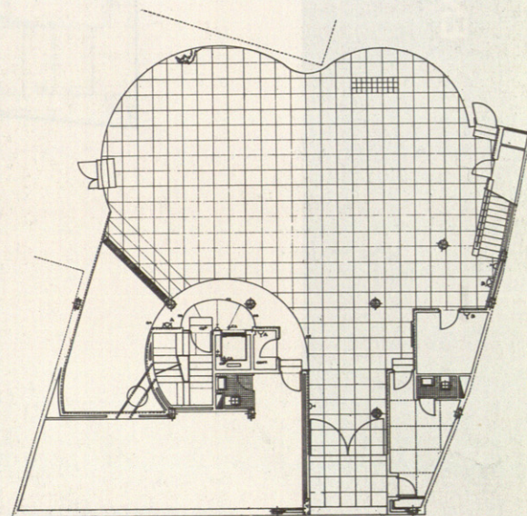
Planta baja. Acceso.
