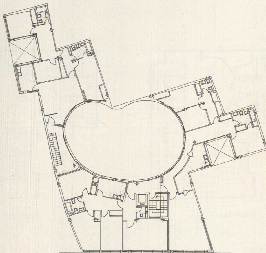
Planta tipo.
