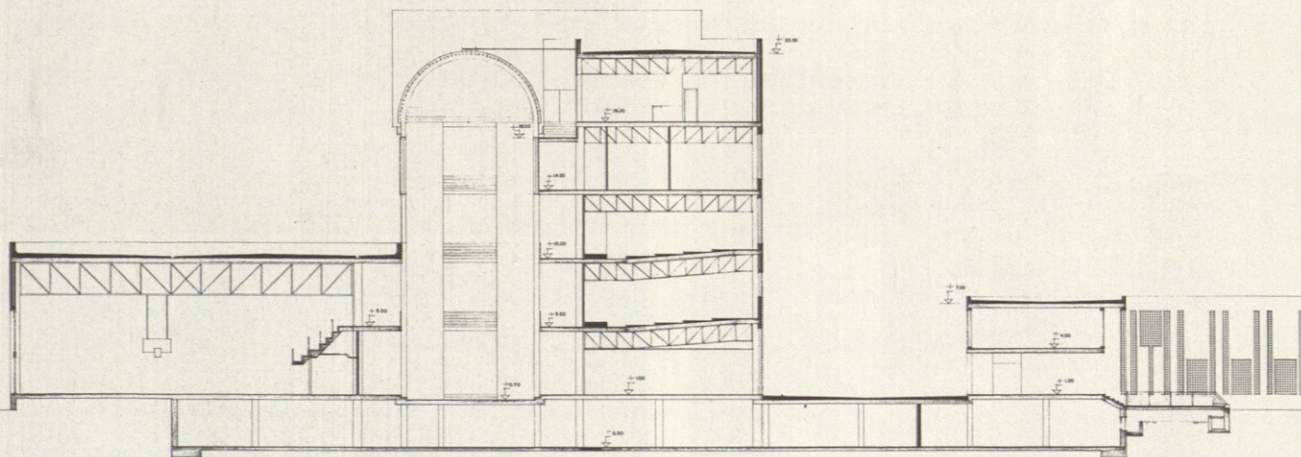
SECCION H.H.
